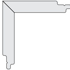
Mitre Corner Detail
